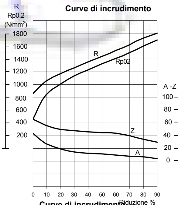
Curve di incrudimento
